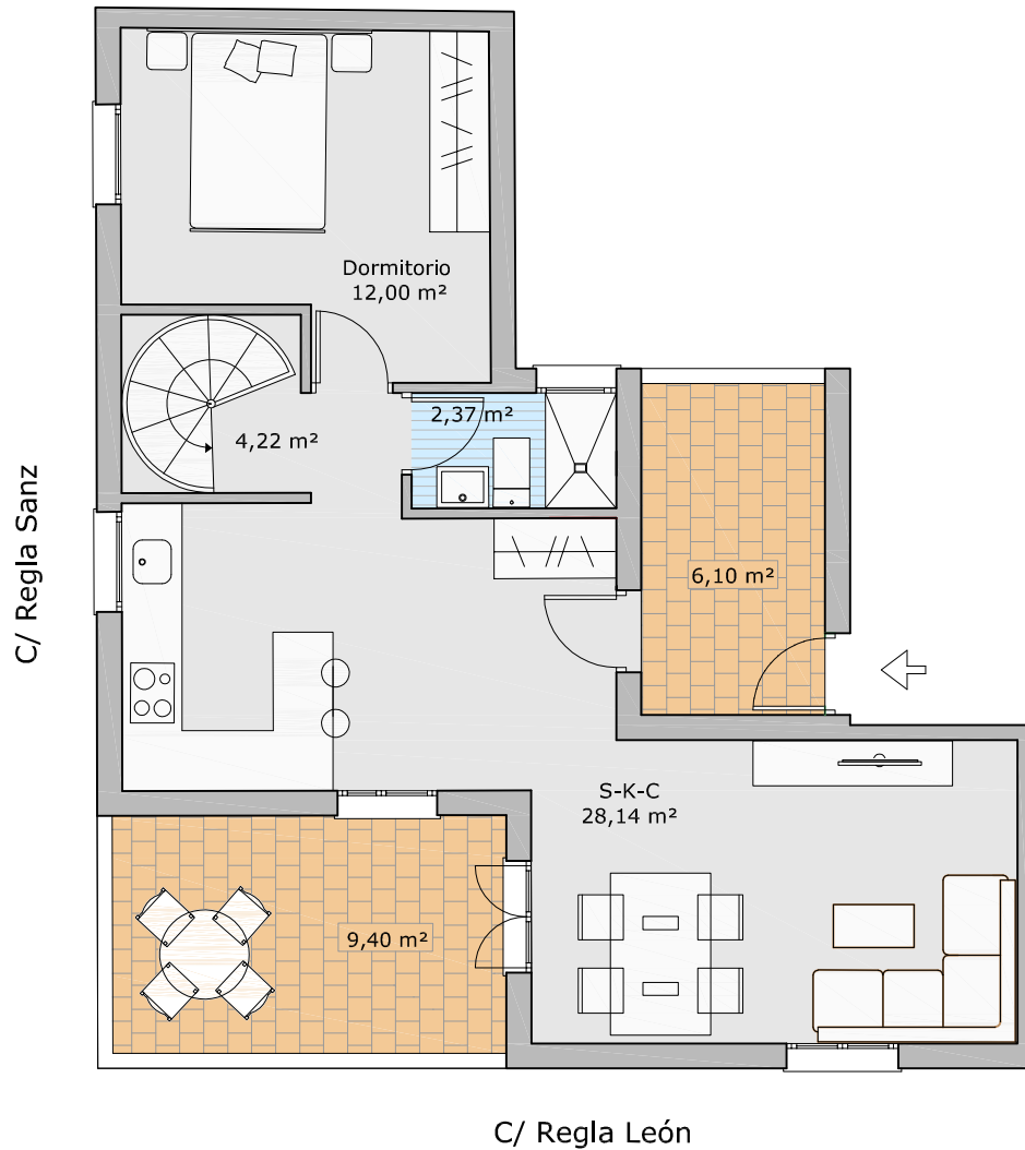
Planta ATICO
