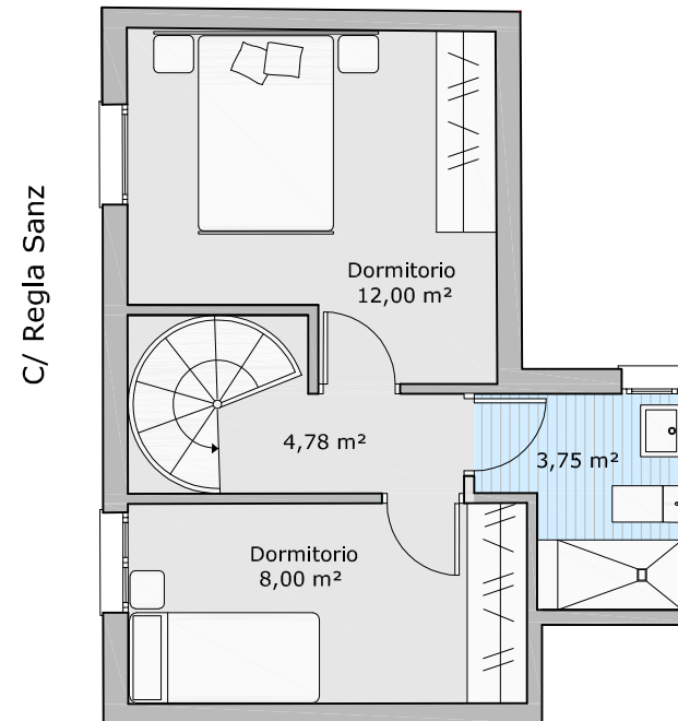
Planta 1ª
